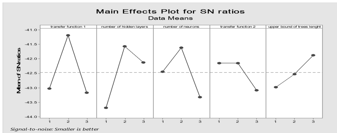
شکل (۲). مقدار پارامتر نرخ سیگنال به نویز خروجی روش تاگوچی
